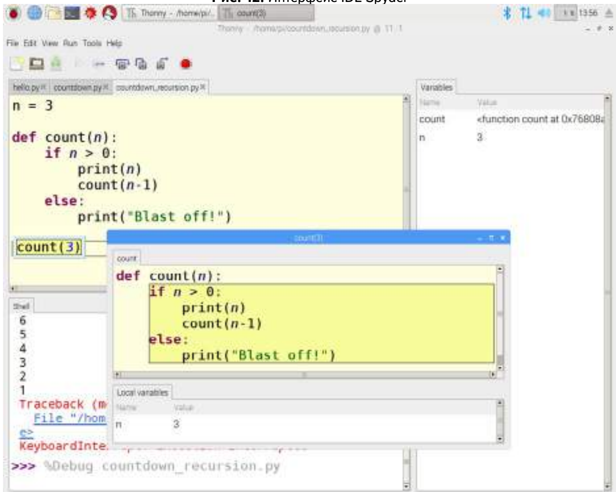
Рис. 13. Интерфейс IDE Thonny
